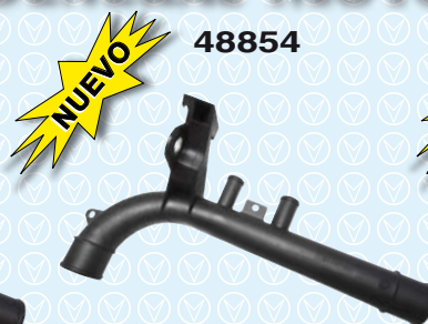
NUEVO 48854 No. Original 90448854 Tubo de Enfriamiento GM Chevy 1.4L y 1.6L 96-07
