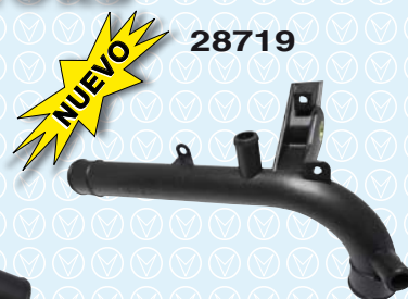
NUEVO 28719 No. Original 9128719 Tubo de Enfriamiento GM Corsa 1.4L (Español), 1.8L (Brasil) Meriva (todos) Astra 02-08, Turbo Tornado s/aire 03-05
